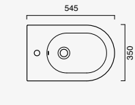
Sfera Bidet 54x35 cod. 1BSF5400
