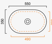
Sfera 55x35 cod. 155ASF00
