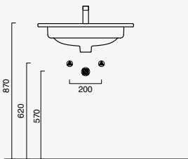
Sfera 45x34 cod. 145BSF00
