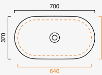
Sfera 70x37 cod. 170ASF00
