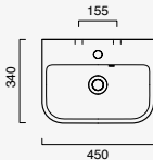
Sfera 45x34 cod. 145BSF00
