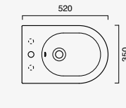
Sfera Bidet 52x35 cod. 1BIC5200
