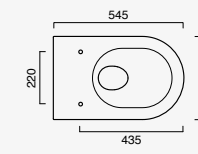
Sfera Wc 54x35 cod. 1VSF54A00
