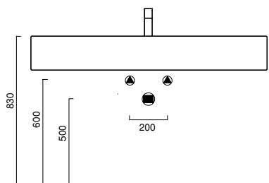
Sistema VERSO - LAVABO 120 / 120 WASHBASIN / WASCHTISCH 120 - 12VE - Kg. 40
