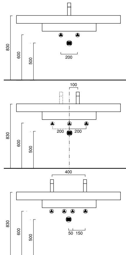
Sistema ZERODomino - LAVABO 125 / 125 WASHBASIN / WASCHTISCH 125 - 125DO - Kg. 36
