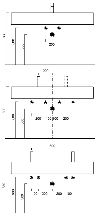
Sistema VERSO - LAVABO 120 / WASH BASIN 120 / WASCHTISCH 120 - 12VE - Kg. 40
